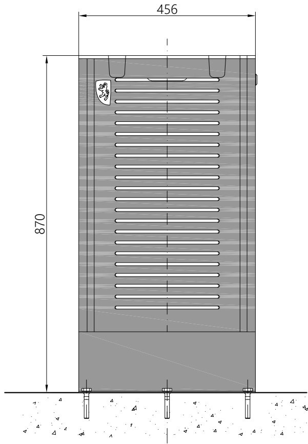
ALZADO FRONTAL
